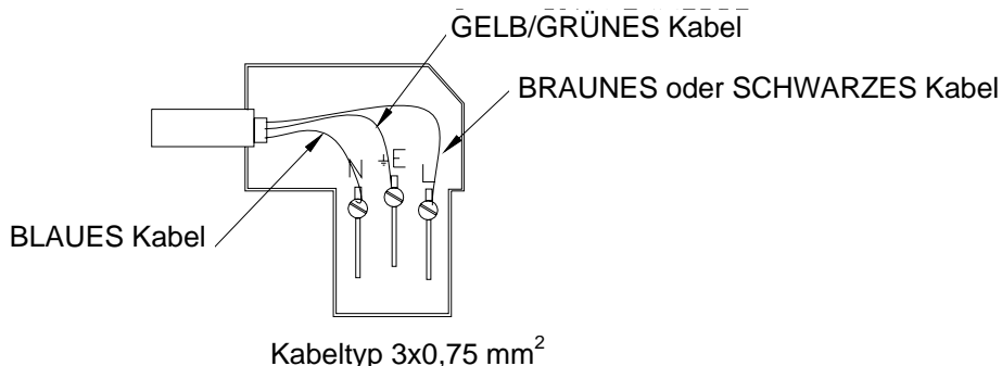
Abbildung 14 – Verkabelung des dreipoligen Steckers
