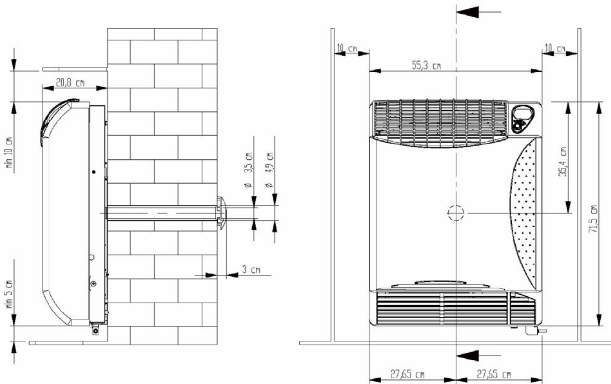
Abbildung 1 – Abmessungen der Heizkörper Calorio
